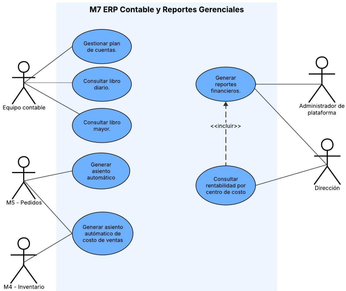
Figura 1. Diagrama de casos de uso del módulo 7(M7)
